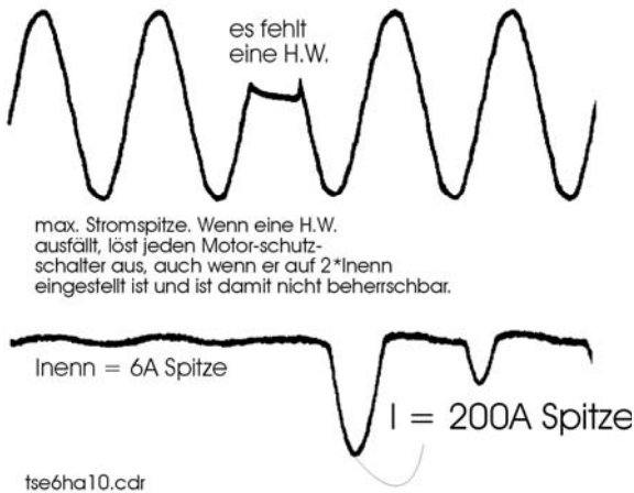
Bild 1. Halbwellenausfall-Simulation an einem geschweißten 1kVA EI Trafo mit 1 kW belastet. (weicher Trafo)
